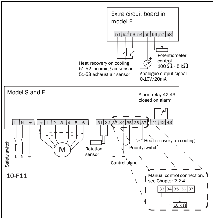
Fig. 6 Wiring diagram
